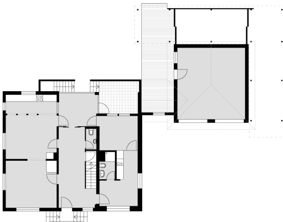
Grundriss Erdgeschoss
